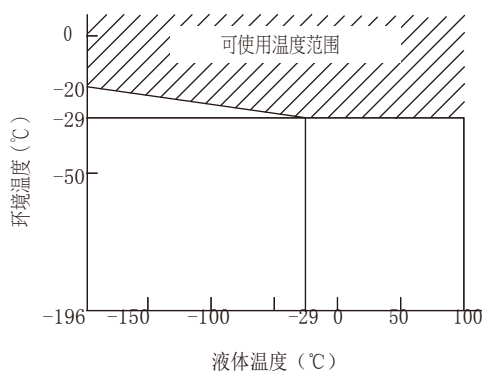
图5 低温型流体温度范围
