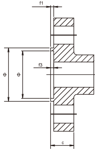
密封面结构
