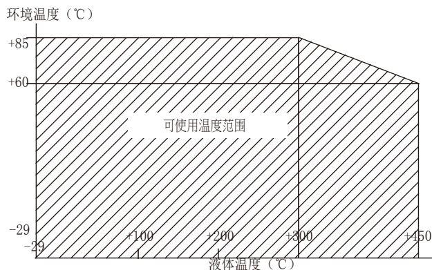
图4 高温型流体温度范围 (一体型)
